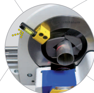
❖ Встроенный лазер
